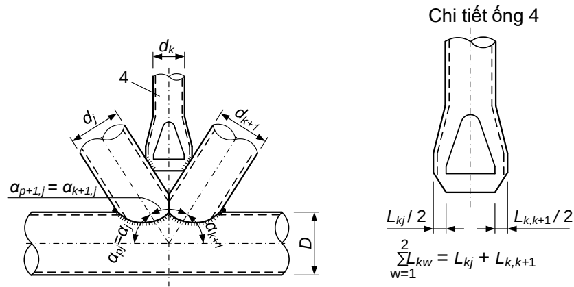
b) Ba thanh bụng (có bóp bụng đầu thanh đứng) giao nhau
