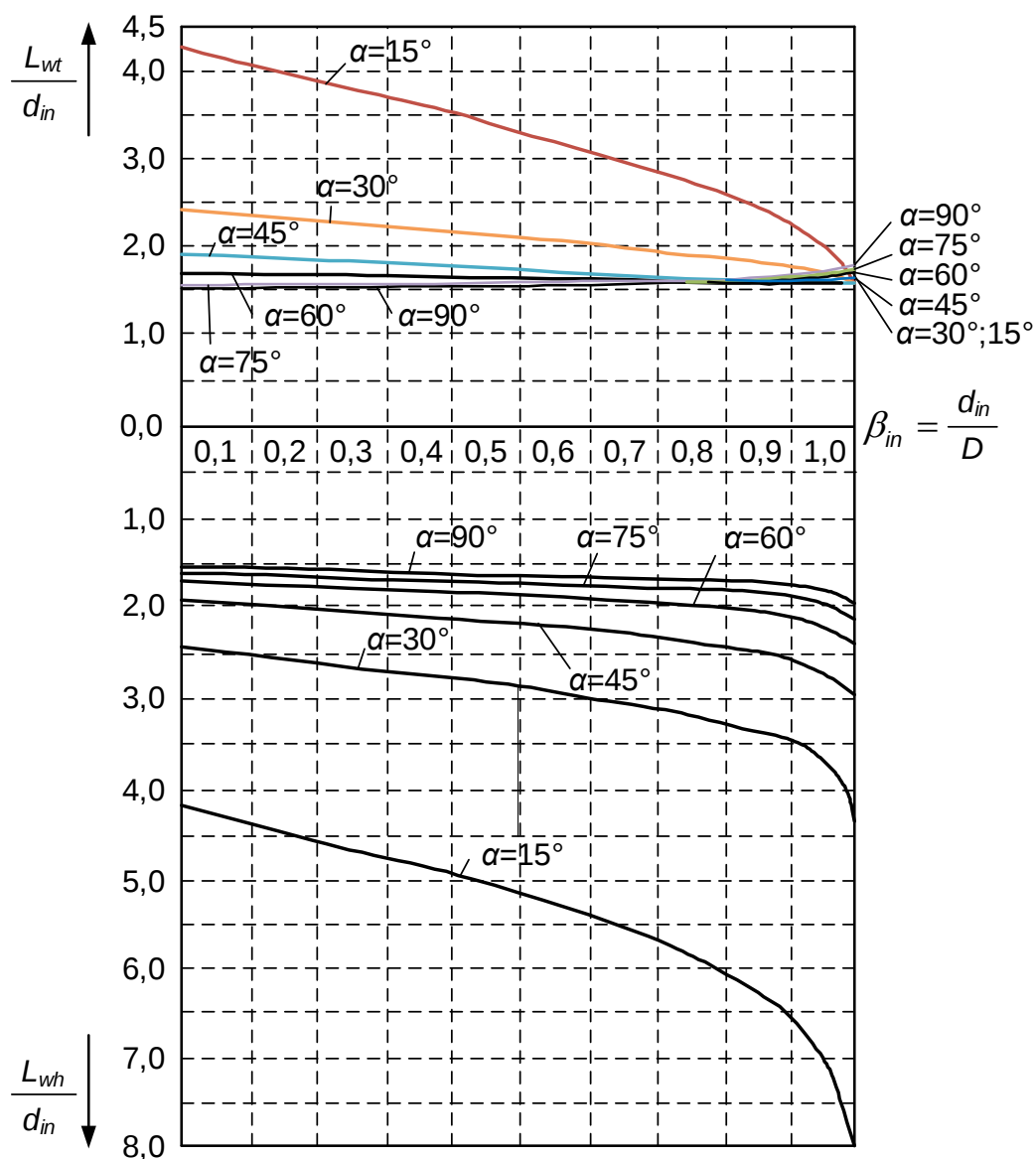
Hình I.10 – Các đồ thị để xác định tổng chiều dài đoạn đường hàn gót L_{wt} và tổng chiều dài đoạn đường hàn mũi L_{wh} trong liên kết hai ống thép
