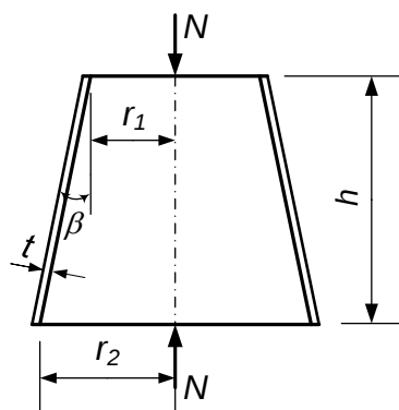
Hình 20 – Sơ đồ vỏ nón tròn xoay chịu lực nén dọc trục
